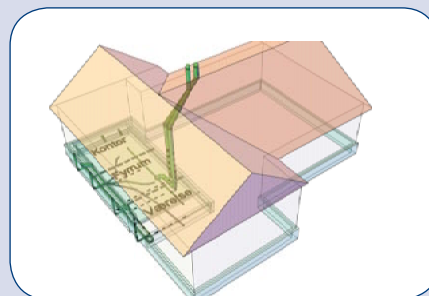
Indeklimasikring ved ventilering under gulv
